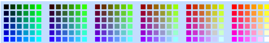
Abbildung 25.3.3.4.2: Web-Farb-Palette
