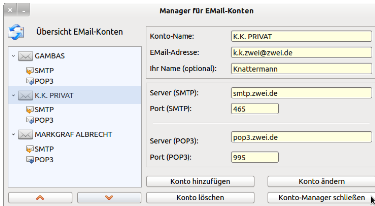
Abbildung 24.3.4.1: GUI: EMail-Konto-Manager
