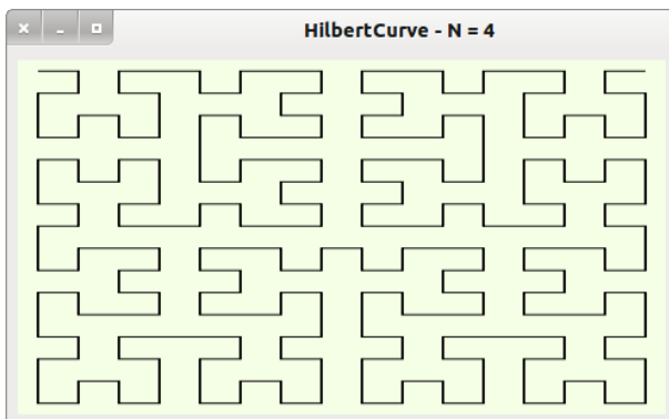
Abbildung 23.3.5.0.1: Fraktal – Hilbert-Kurve
